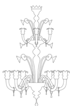
7653/6+3 Ø 85 cm H. 120 cm 20 kg 0,26 mc E 14 led
