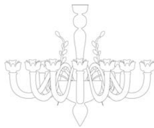
7998/10 Ø 105 cm H. 90 cm 24 kg 0,40 mc E 14 led
