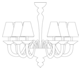
7779/10 Ø 110 cm H. 85 cm 15 kg 0,26 mc E 14 led
