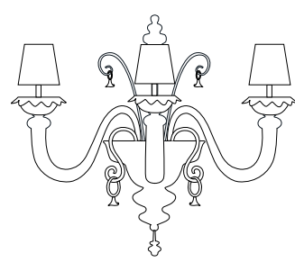
8047P/A3 L30x25 cm H. 55 cm 6 kg 0,12 mc E 14 led
