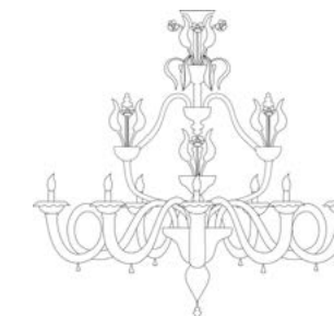
7778/8 L. 140x110 cm H. 125 cm 50 kg 0,65 mc E 14 led
