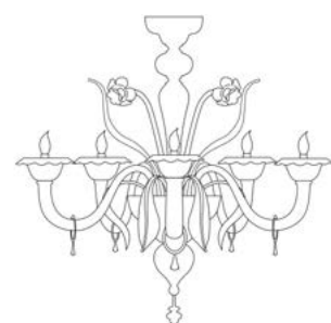
7413/6 Ø 82 cm H. 80 cm 16 kg 0,20 mc E 14 led
