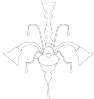
7865/3 Ø 62 cm H. 70 cm 10 kg 0,12 mc E 14 led
