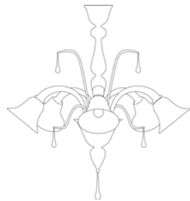
7865/5 Ø 85 cm H. 80 cm 12 kg 0,20 mc E 14 led
