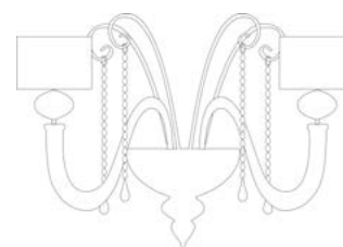
7872/A2 L. 25x25 cm H. 45 cm 5 kg 0,12 mc E 14 led
