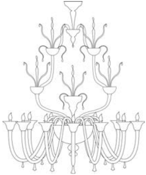
7923/12 Ø 163 cm H. 150 cm 80 kg 1,00 mc E 14 led
